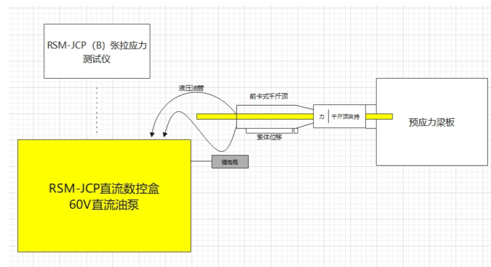
图2-2 RSM-JCP(B)张拉应力测试仪现场连接示意图
