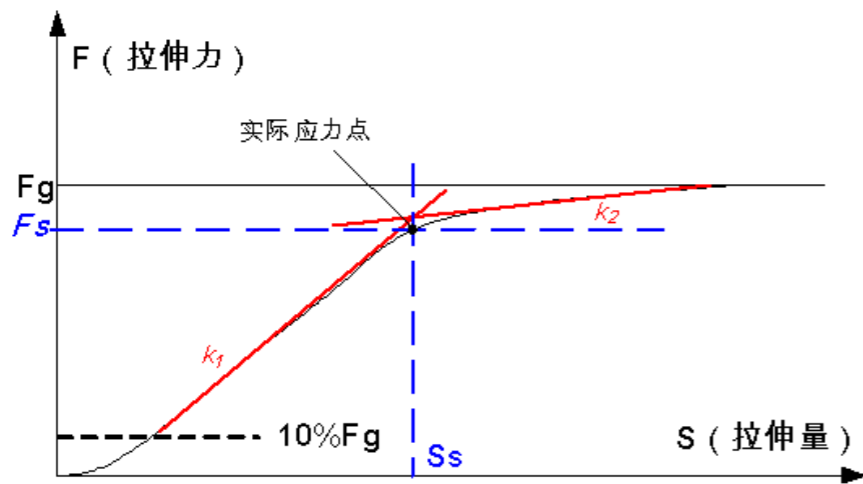
图2-3 RSM-JCP(B)张拉应力测试仪测试原理图
