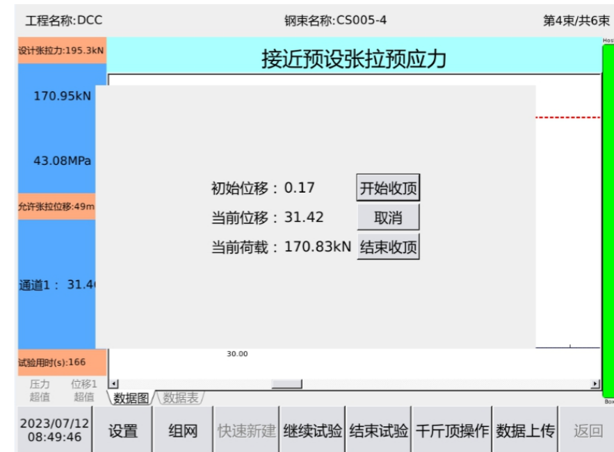
图3-3 (r) 试验引导-收顶界面
