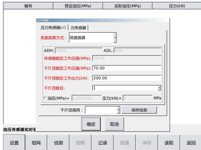
图5-7 千斤顶设置界面
