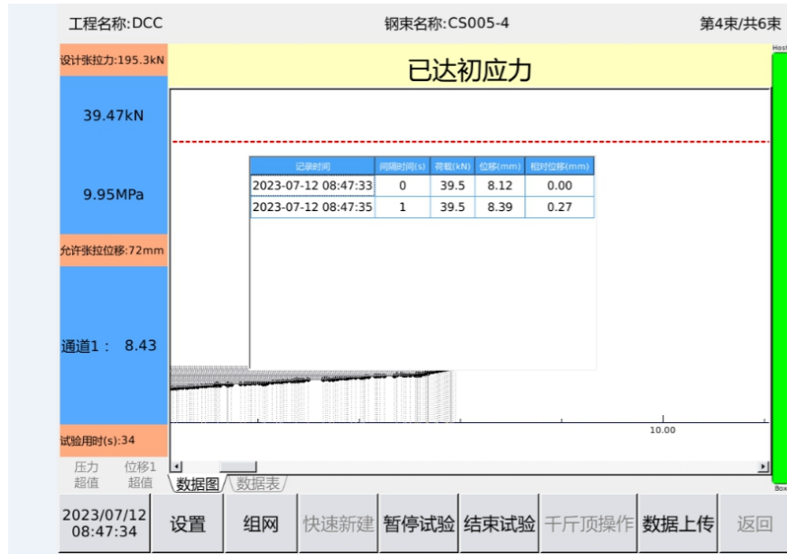
图3-3 (m) 试验引导-初应力维荷示意图
