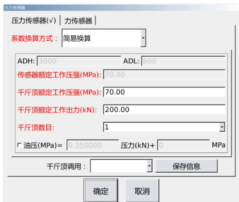
图3-5 (e) 压力传感器标定设置界面图
