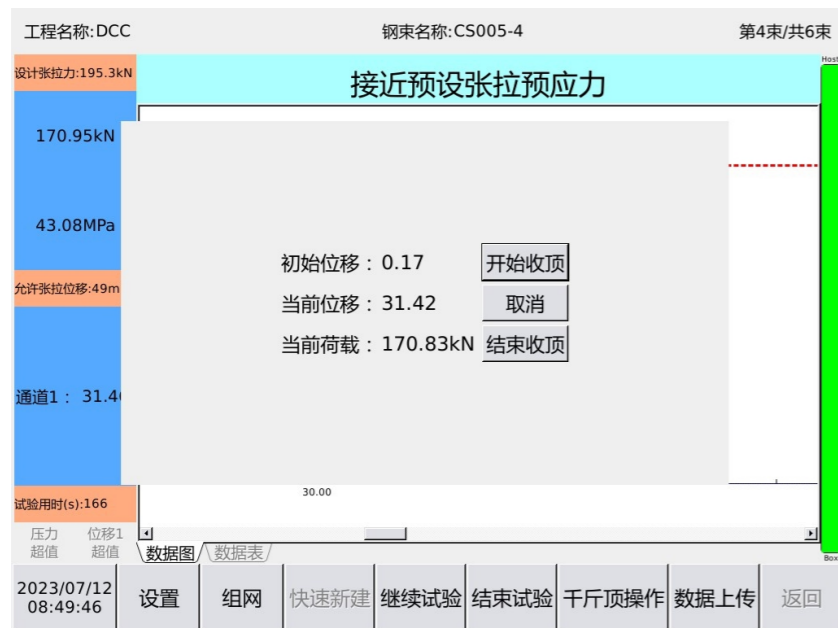
图5-13 收千斤顶界面
