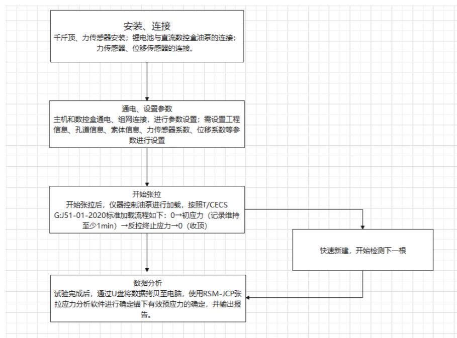
图2-4 RSM-JCP(B)张拉应力测试仪现场测试流程图
