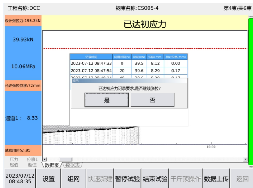
图3-3 (n) 试验引导-初应力达到维荷要求示意图
