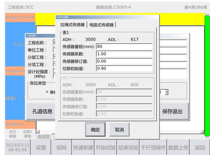
图5-8 位移传感器设置界面
