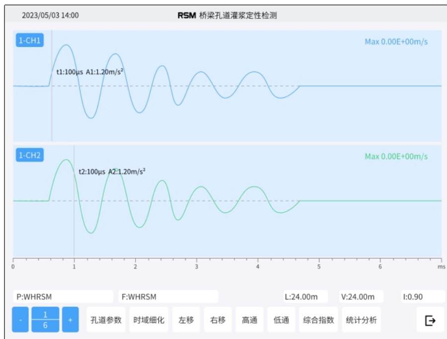
图4-4 定性检测分析界面
