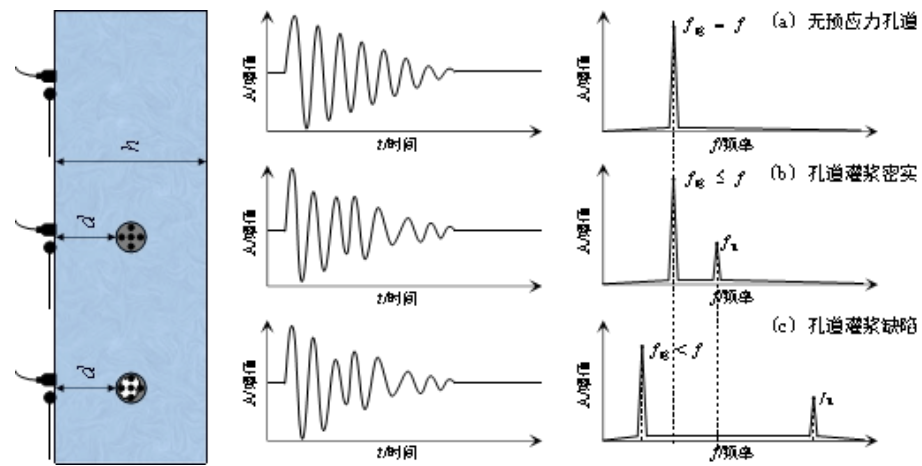
图5-10 灌浆质量检测分析示意图
