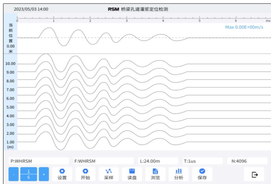
图4-5 定位检测采集主界面
