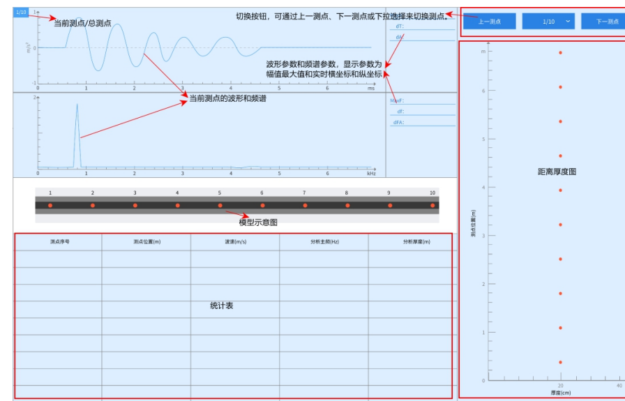
图5-7 分析视图
