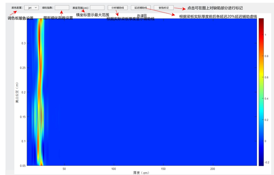
图5-8 结果展示
