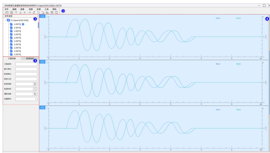
图5-1 软件主界面
