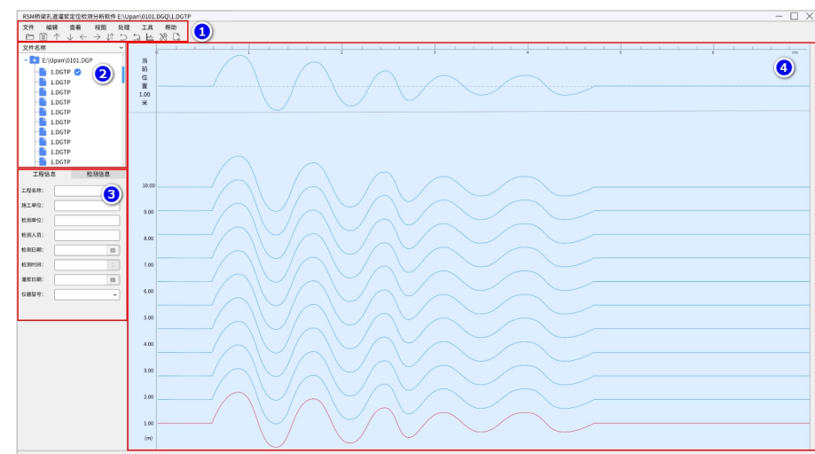
图5-1 软件主界面
