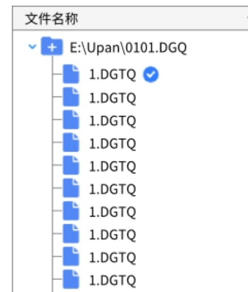
图5-3 文件列表
