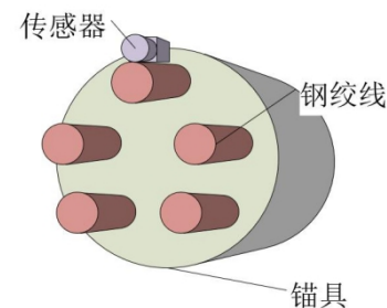
图4-8 传感器安装示意图
