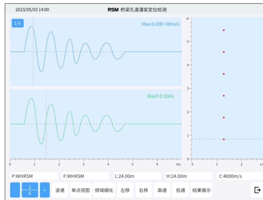
图4-7 定位检测分析界面
