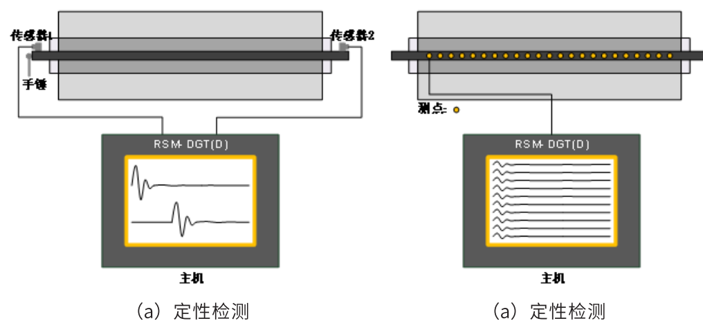
图3-1 桥梁孔道灌浆质量检测仪基本原理
