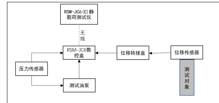
图2-2 (a) RSM-JC6(C)静载荷测试仪 (有线位移) 示意图
