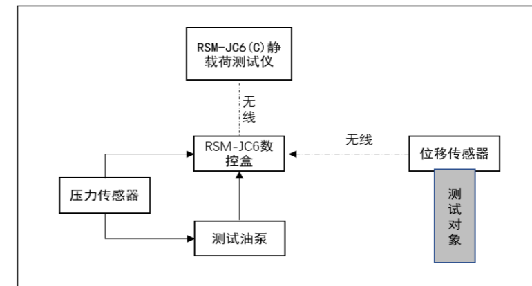
图2-2 (b) RSM-JC6(C)静载荷测试仪 (无线位移) 示意图
