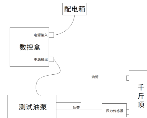
图2-3 RSM-JC6(C)静载荷测试仪 (无线位移) 示意图
