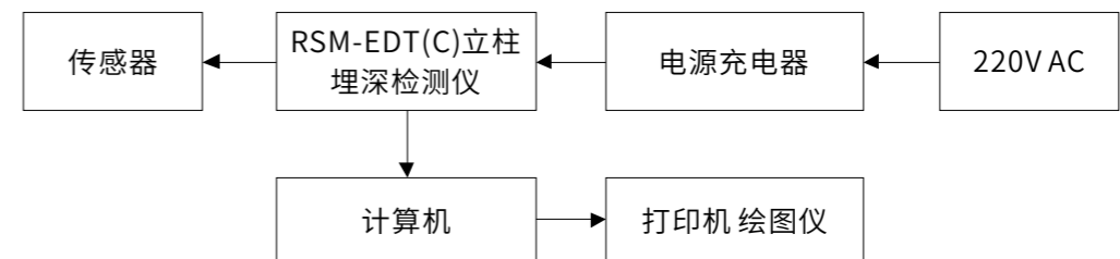
图2-4 立柱埋深检测外围设备示意图
