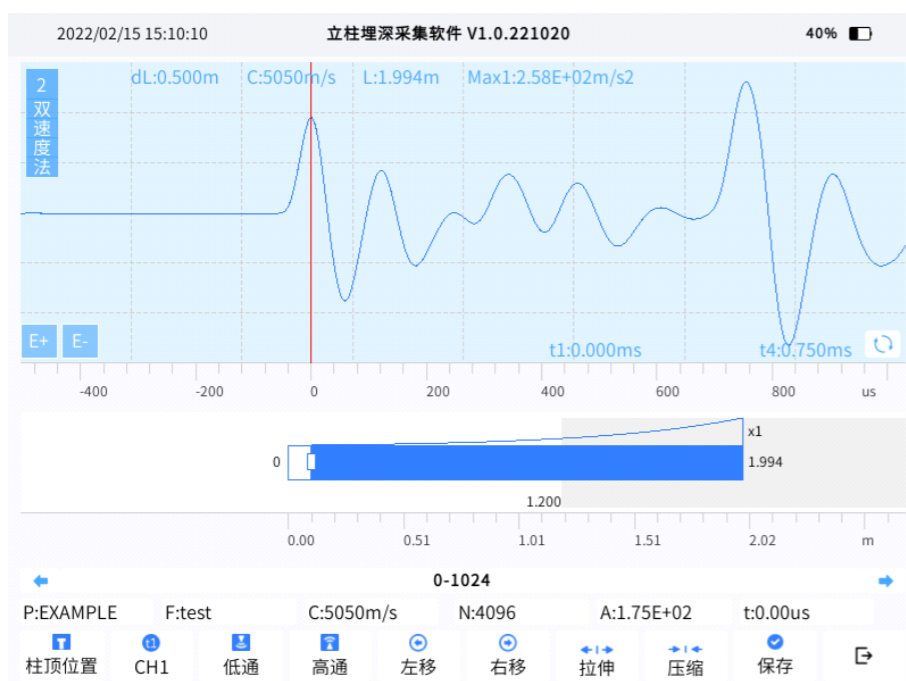
图4-19 反算界面
