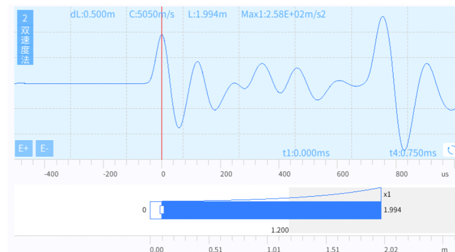
图4-21 波形分析区
