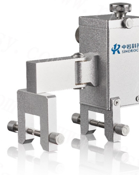
图2-3 RSM-CS1可控激振器
