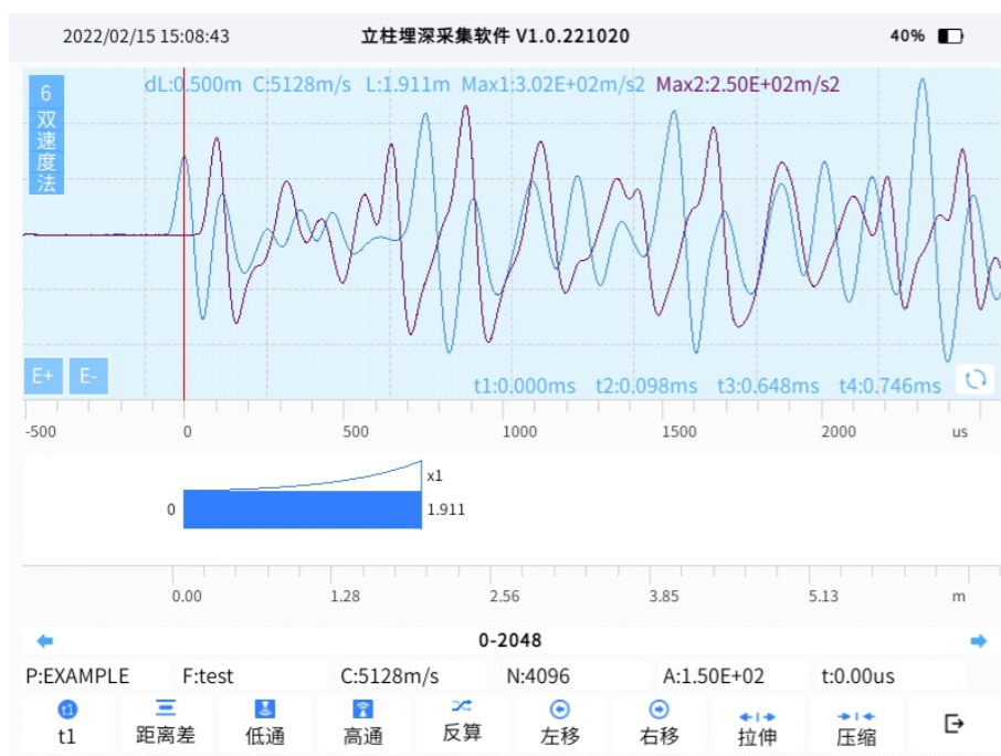
图4-16 波形分析区
