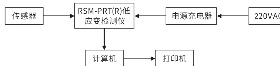
图2-3 RSM-PRT(R)基桩低应变检测系统示意图
