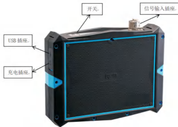
图2-2 RSM-PRT(R)基桩低应变检测仪各接口示意图
