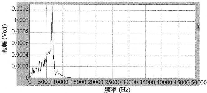
图3 边界影响区域外的测试结果
