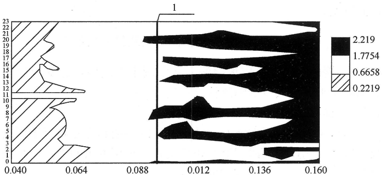
图 10 滑移后检测区域不同深度的相对振幅（时间——距离）示意图
