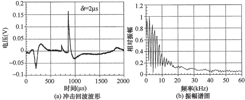
图 7 无效的冲击回波检测示图
