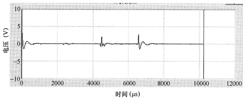
图 13 典型结合面完好冲击回波时程图
