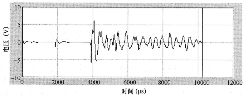
图 12 典型结合面空鼓冲击回波时程图
