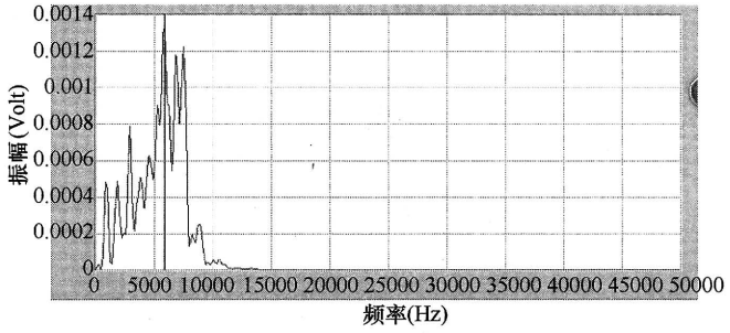
图 4 边界影响区域内的测试结果
